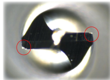
Standard-Bohrer 10 Bohrungen Starker Verschleiß
