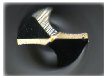
DIXI 1137 DRYCUT 900 Bohrungen Kein Verschleiß
