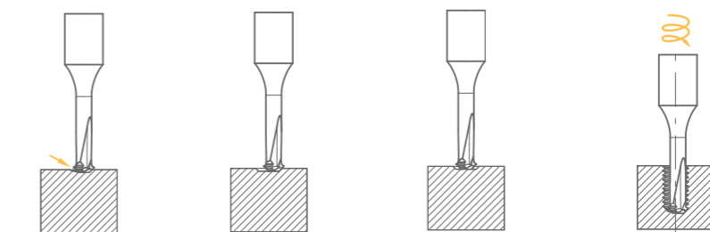
1 Spil starten Verplaatsen naar X0Y0Z0.10 2 360° Circulaire interpolatie 3 Terug naar het middelpunt X0 Y0 4 Circulaire boor-draadrees. Frees naar het middelpunt draadgat bij einde cyclus.
