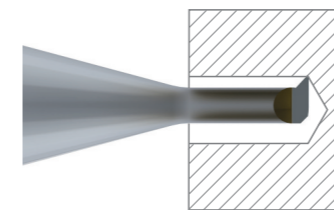
Alesatura per foro cieco
