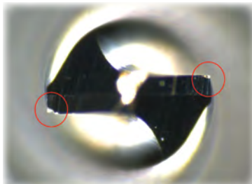
Usura pronunciata Materiale che si attacca al centro dell'utensile
