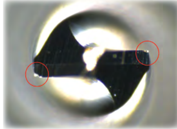
Starker Verschleiß Anhaften von Material in der Mitte des Werkzeugs
